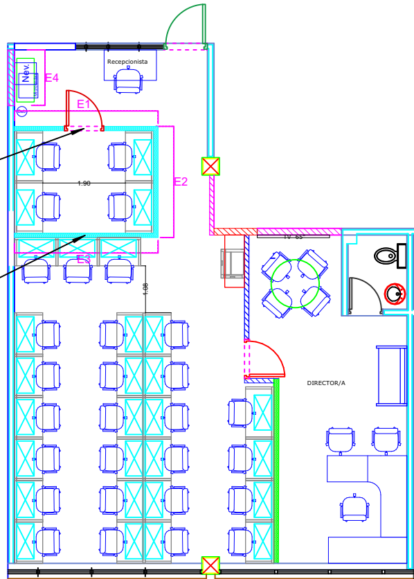
Planta Arquitectónica Propuesta
