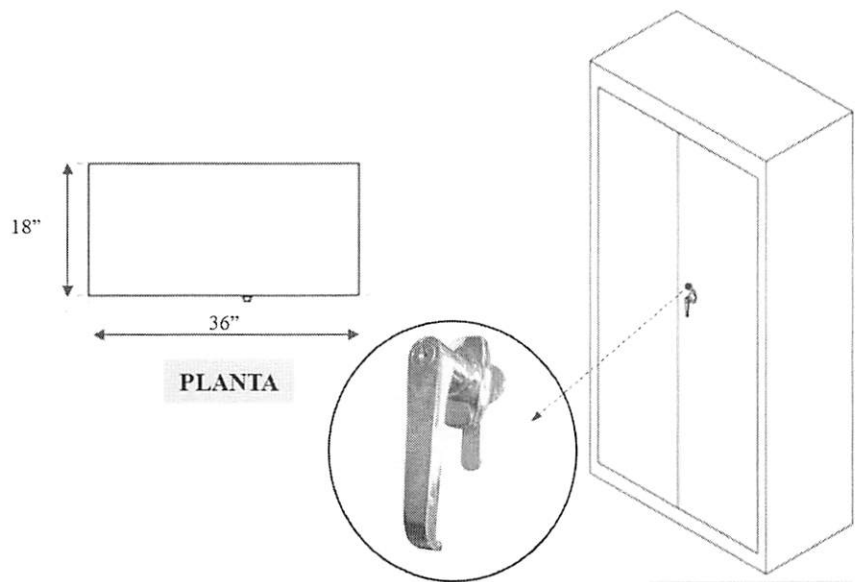
PERSPECTIVA
