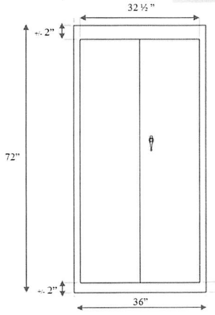
ELEVACION FRONTAL
