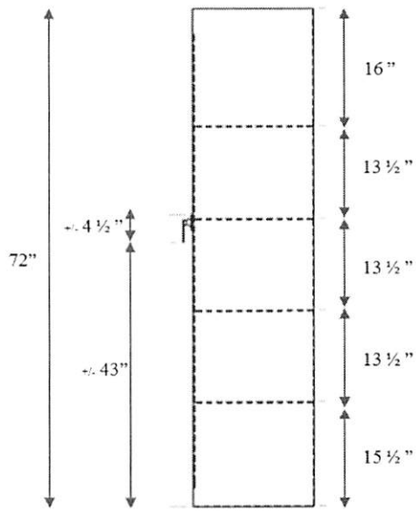
ELEVACION LATERAL
