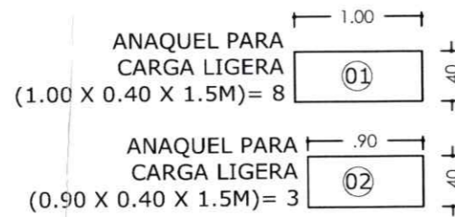
PLANTA ARQUITECTONICA PROPUESTA PRIMER NIVEL FISCALIA SAN CRISTOBAL ESC 1/100
