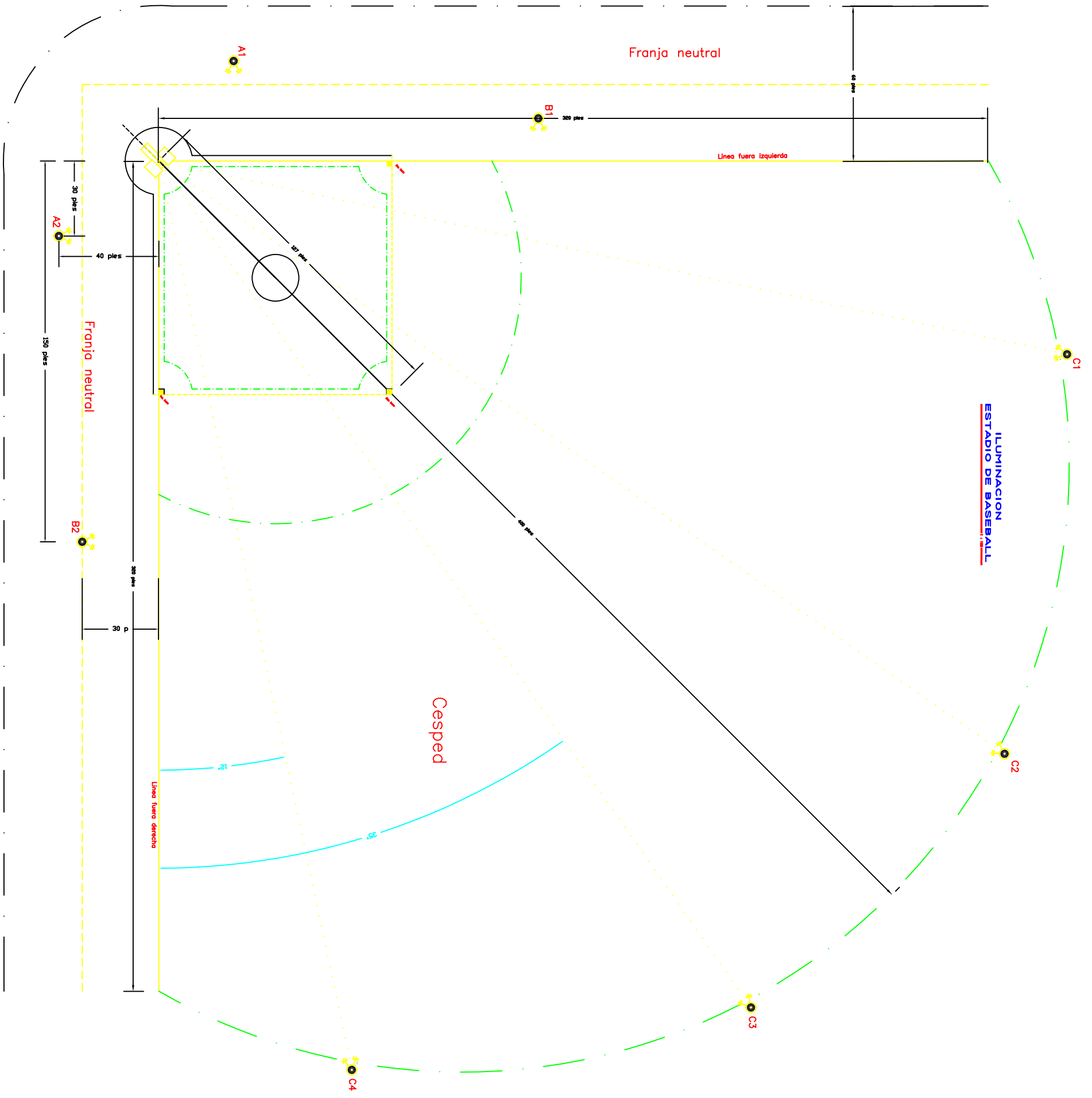
PLANO UBICACION DE POSTES
