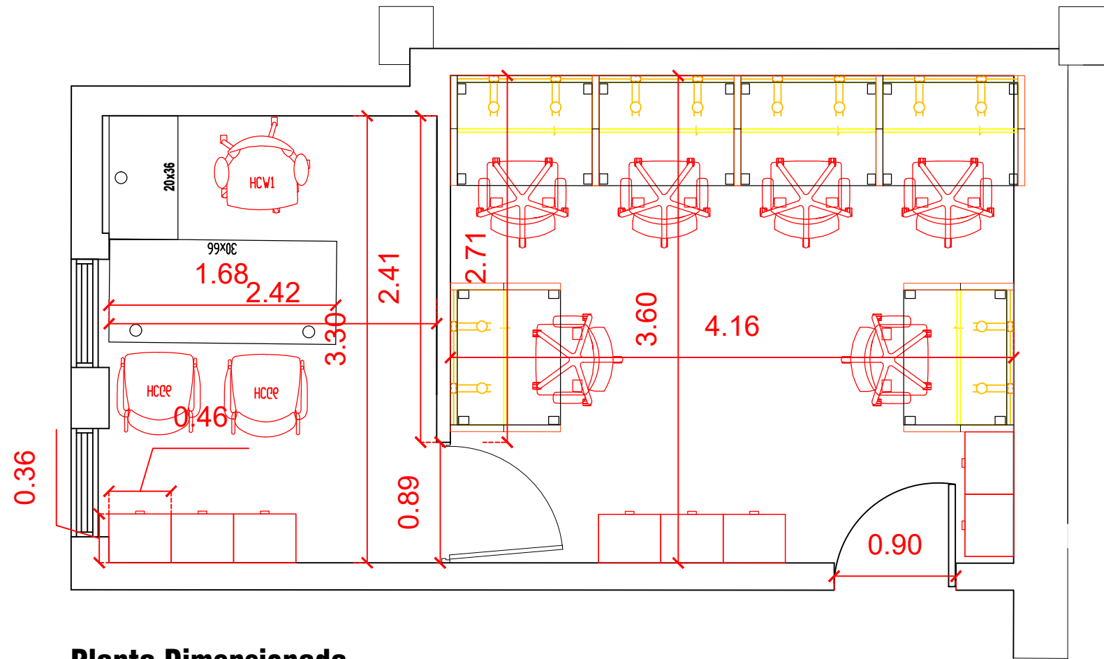
Planta Dimensionada
