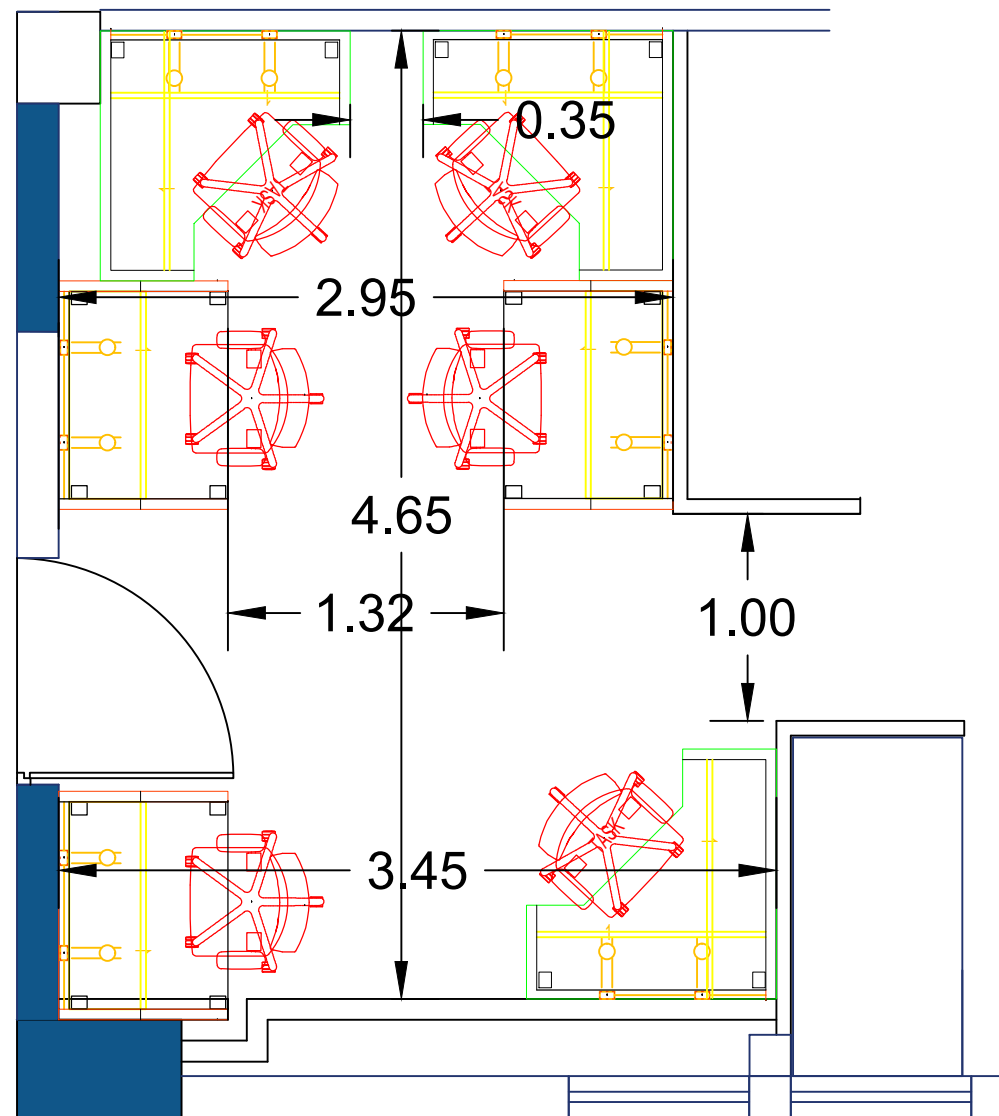
Planta Dimensionada
