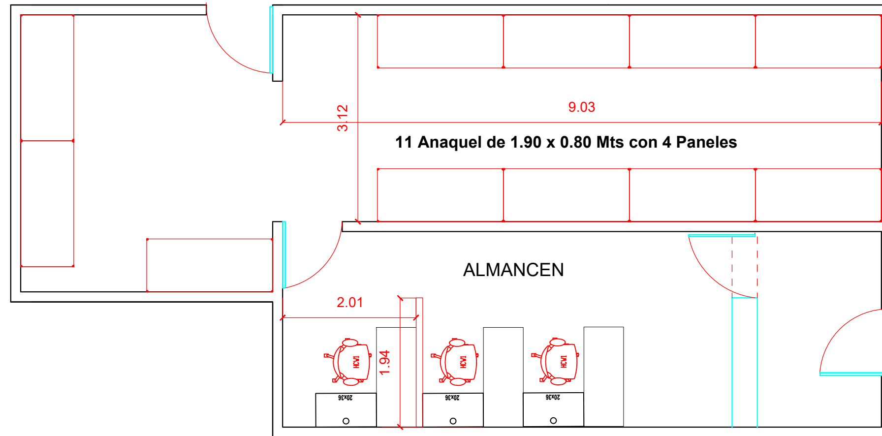
PLANTA DIMENSIONADA ALMACENES Y SUMINISTROS
