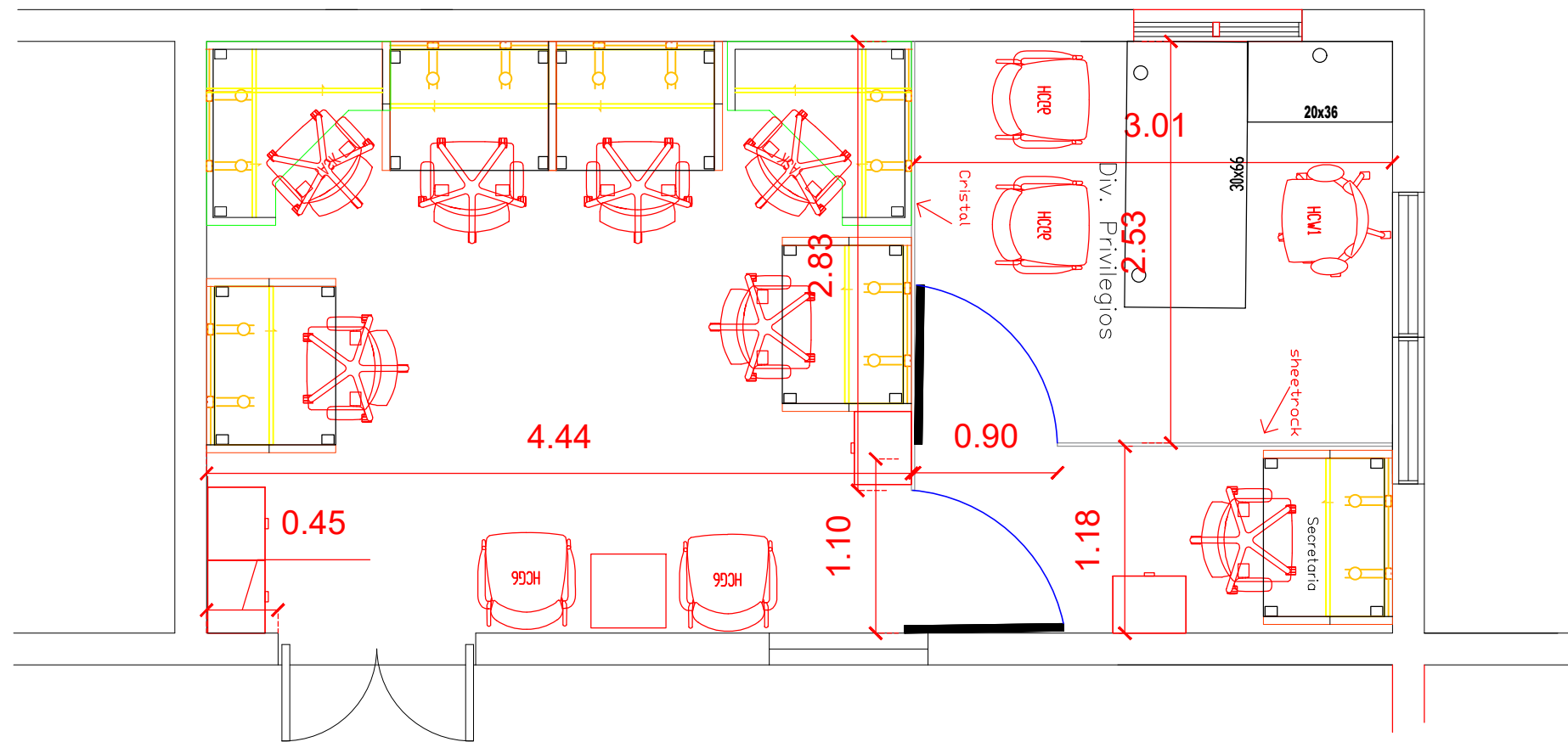
Planta Dimensionada
