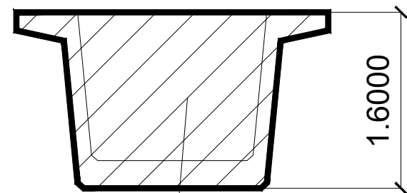
SECCION A-A
