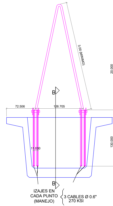
SECCION A-A (IZAJES MANEJO)
