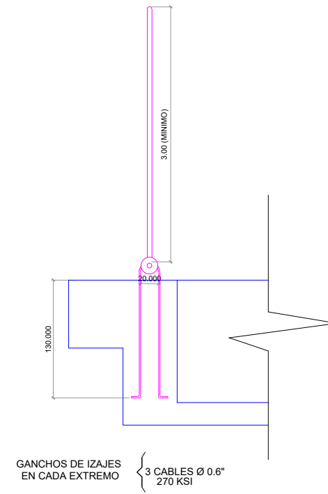
SECCION B-B (IZAJES MANEJO)
