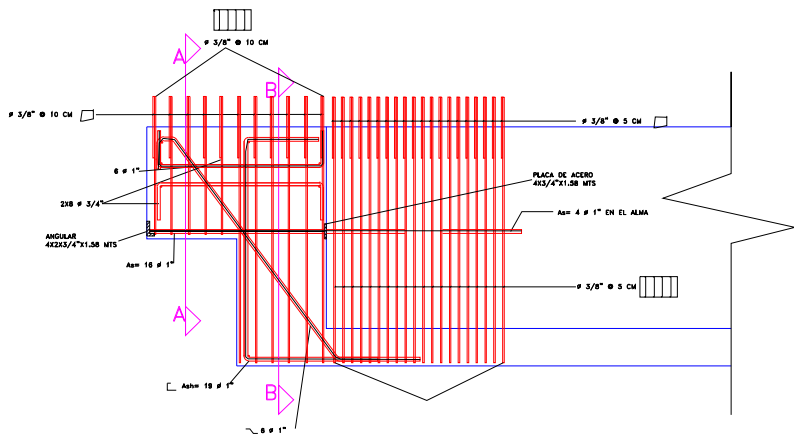
DETALLES DE ARMADO EN EXTREMOS SECCIONES TRANSVERSALES
