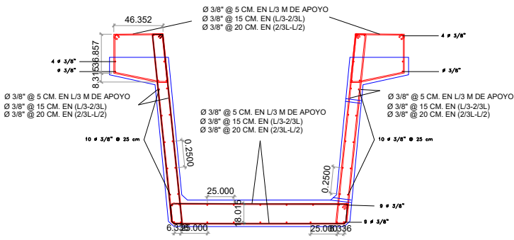
DETALLE DE ARMADO
