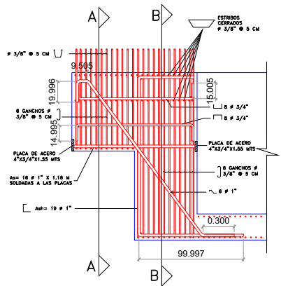
DETALLE DE ARMADO EN EXTREMOS SECCION C-C (EN EL EJE)
