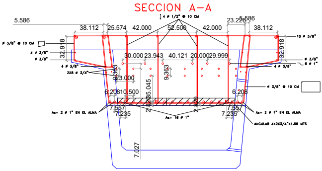
DETALLES DE ARMADO EN EXTREMOS SECCIONES TRANSVERSALES
