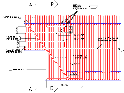
DETALLE DE ARMADO EN EXTREMOS SECCION D-D (EN EL ALMA)
