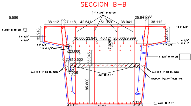
DETALLES DE ARMADO EN EXTREMOS SECCIONES TRANSVERSALES
