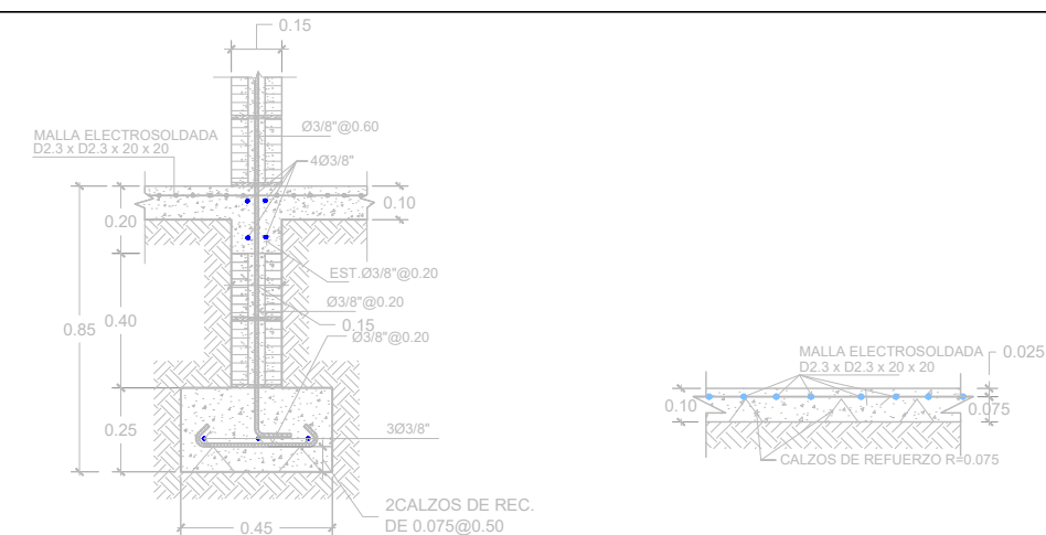
DP DETALLE PISO DE HORMIGON E-01 ESC. 1:15
