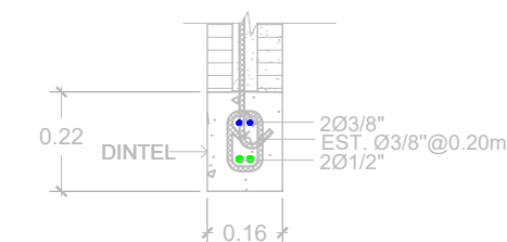
DS1 SECCION (1-1) E-02 ESC. 1:15
