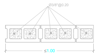
6 DETALLE ARMADO DE MUROS DE LONGITUD IGUAL O MENOR A 1.00 m. E-01 ESC. 1:15
