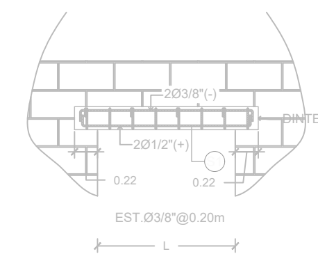
D1 SECCION LONGITUDINAL DINTEL (D1) ESC. 1:40
