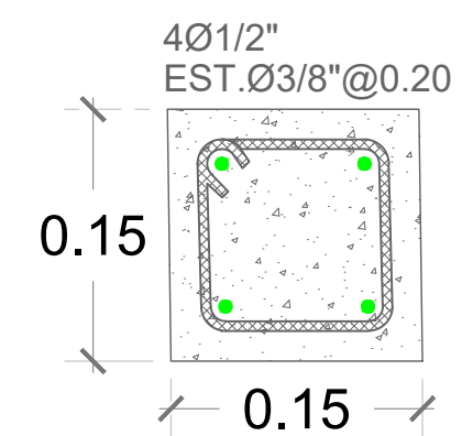
E-02 DETALLE COLUMNA CA ESC. 1:15
