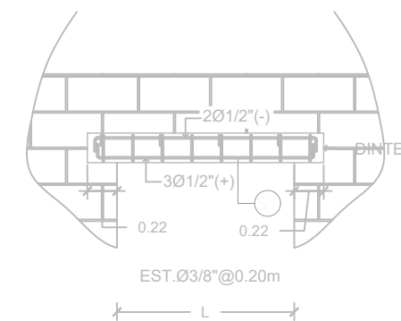
D2 SECCION LONGITUDINAL DINTEL (D2) ESC. 1:40
