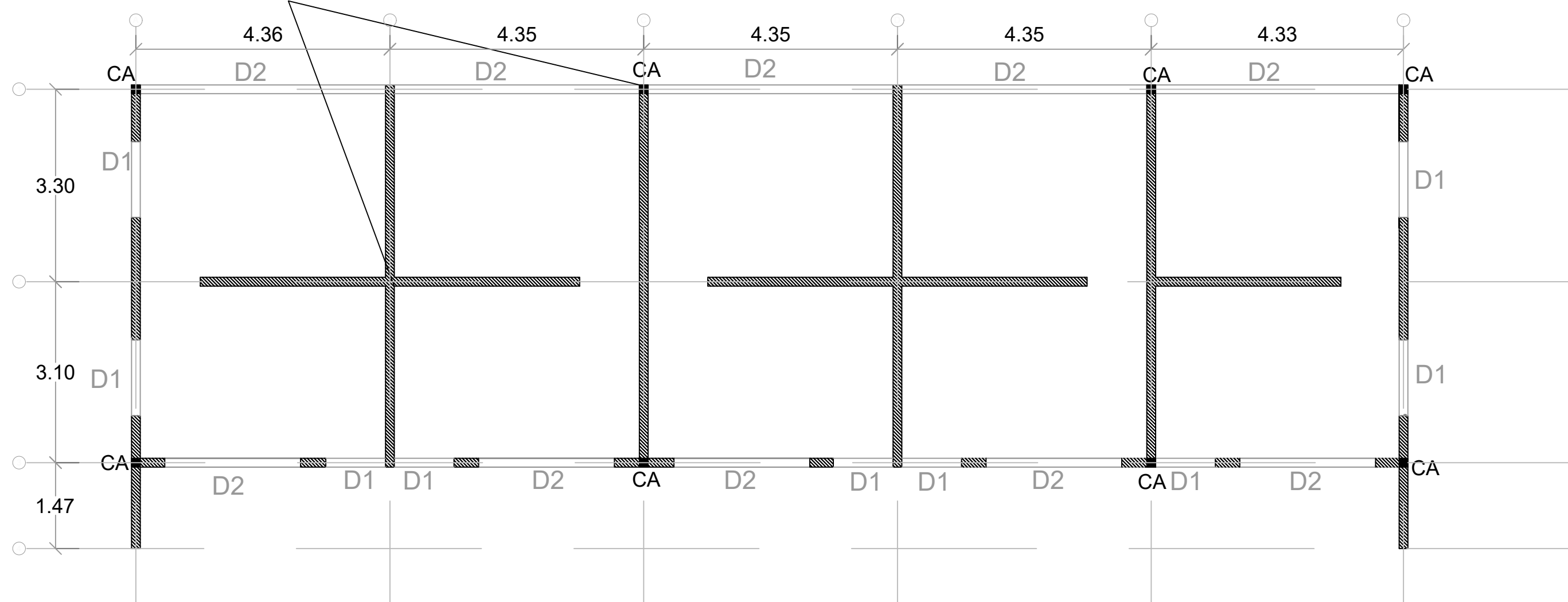
PLANTA DE ENTREPISO ESC. 1:50
