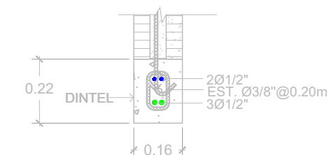
DS1 SECCION (1-1) E-02 ESC. 1:15
