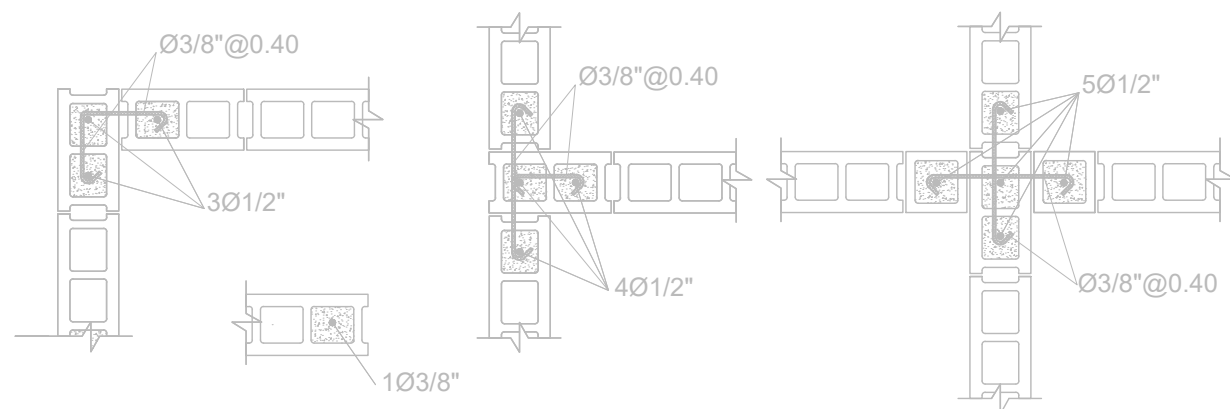
5 DETALLE INTERSECCIONES DE MUROS E-01 ESC. 1:30
