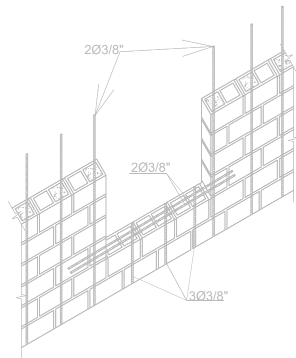
RAV DETALLE REFUERZO ABERTURA VENTANA E-02 ESC. 1:30
