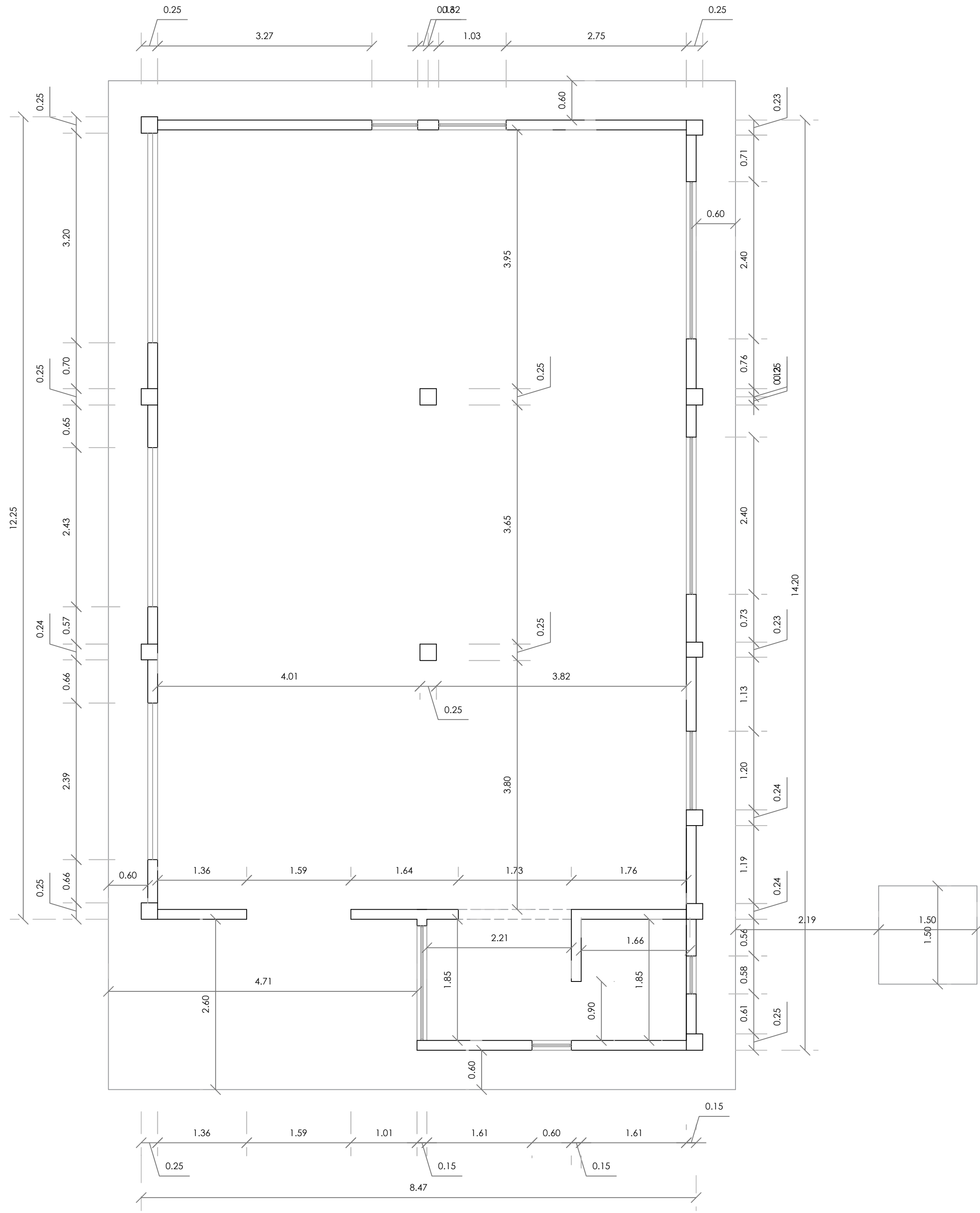
PLANTA DIMENSIONADA LEVANTAMIENTO. DEPÓSITO Escala 1:50
