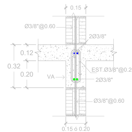
VA VIGA DE AMARRE SNM E-02 ESC. 1:15
