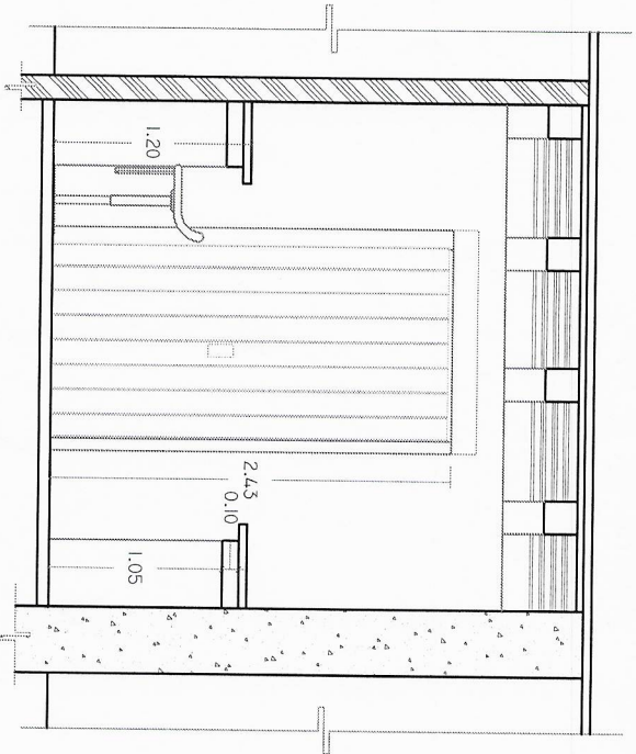
SECCIÓN B-B ESC.: 1:50 MTS.
