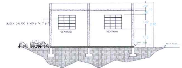
SECCIÓN A-A CASETA
