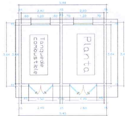
CASETA DIMENSIONADA
