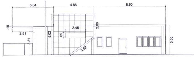
ELEVACION LATERAL DERECHO
