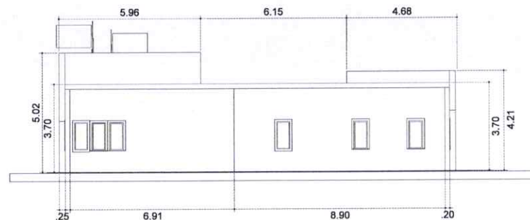
ELEVACION POSTERIOR
