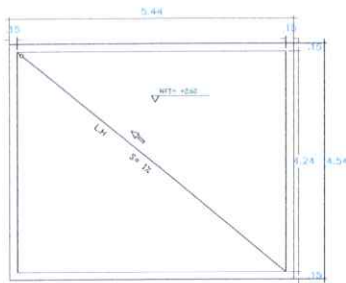
PLANTA DE TECHO
