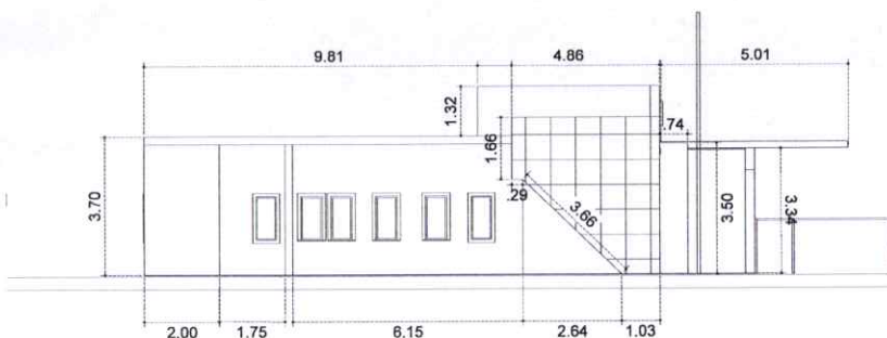
ELEVACION LATERAL IZQUIERDO
