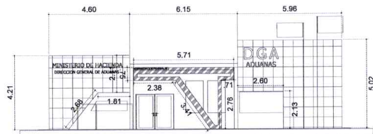
ELEVACION FRONTAL
