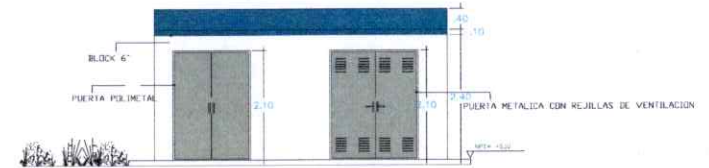
ELEVACIÓN FRONTAL CASETA
