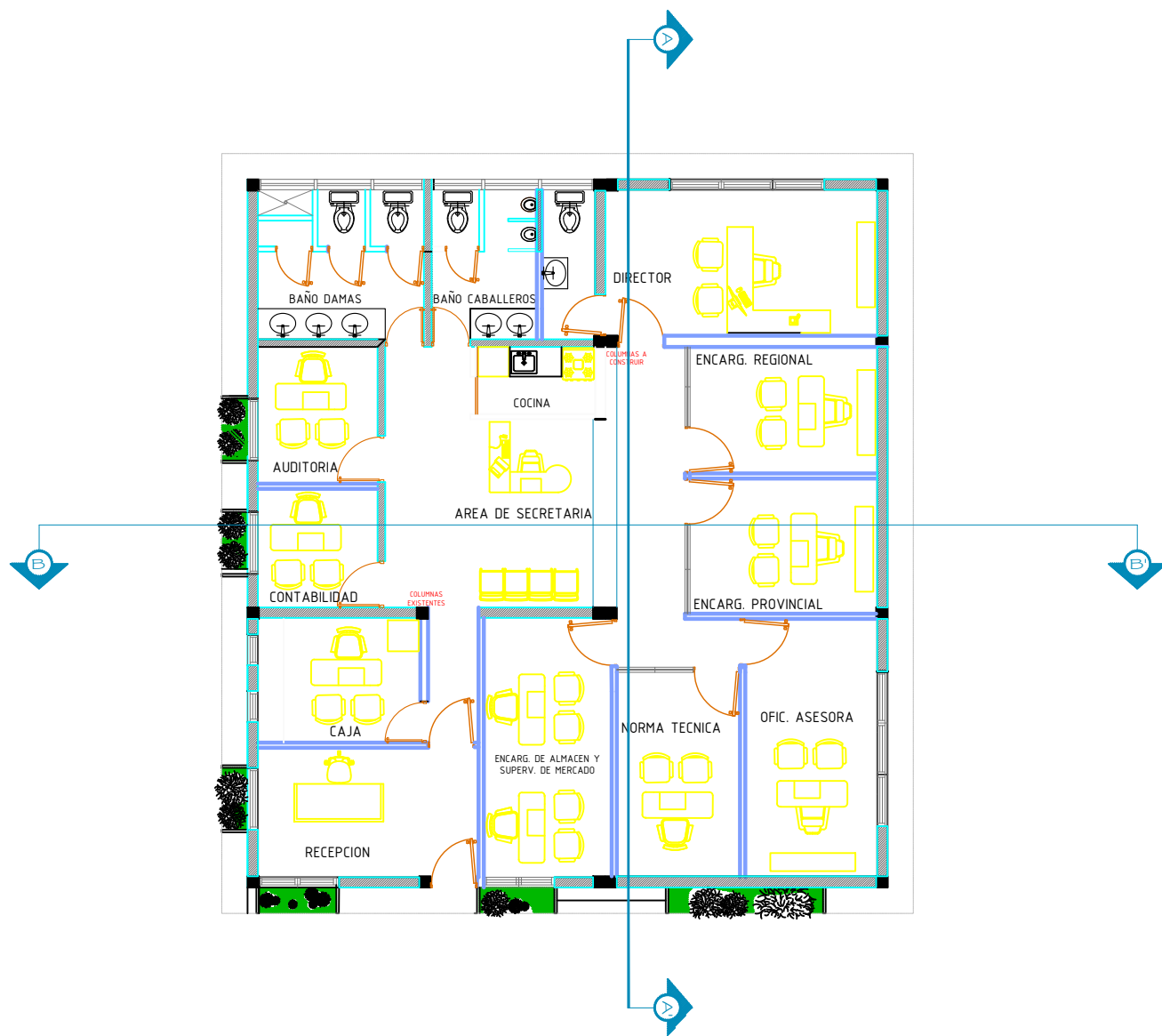
Planta Arquitectónica/Propuesta 0 10 20 30 40 50 100m ESCALA GRAFICA
