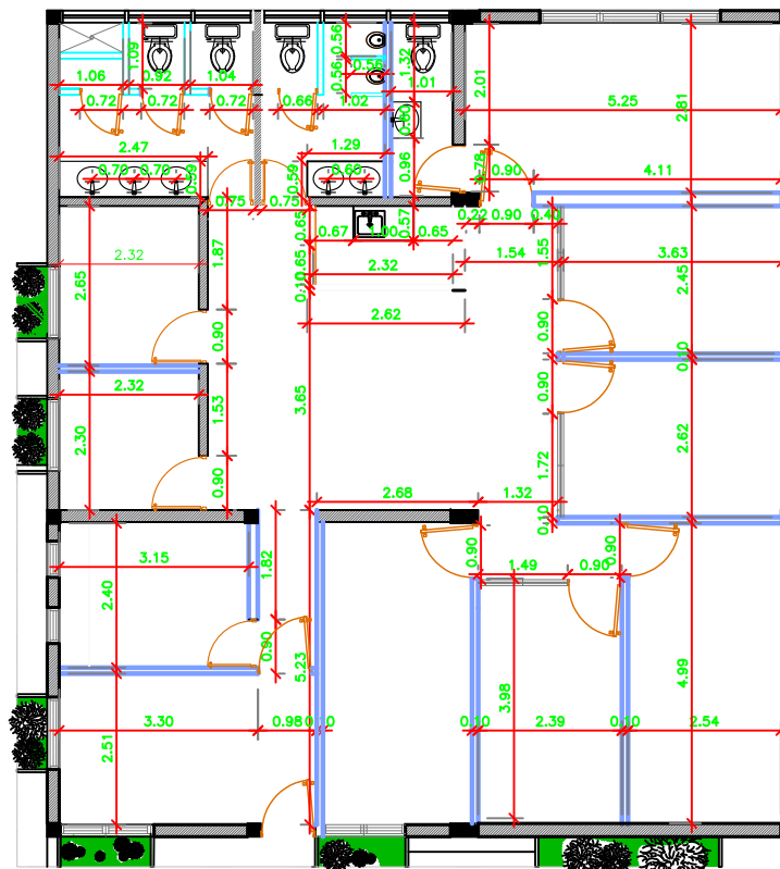
Planta Arquitectónica Dimensionada Propuesta/muros interior
