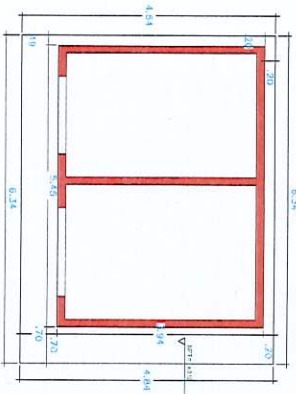
PLATEA DIMENSIONADA
