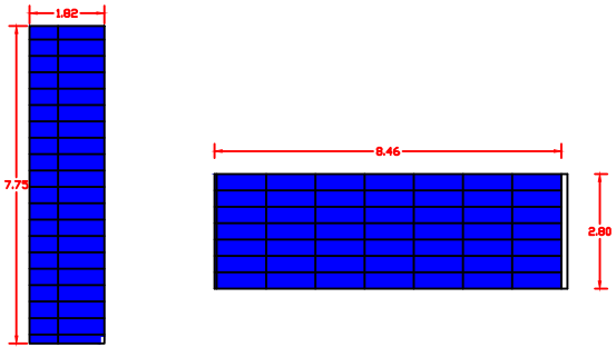
DETALLE DE PROPUESTA DE FACHADA ELEVACION LATERAL IZQ.
