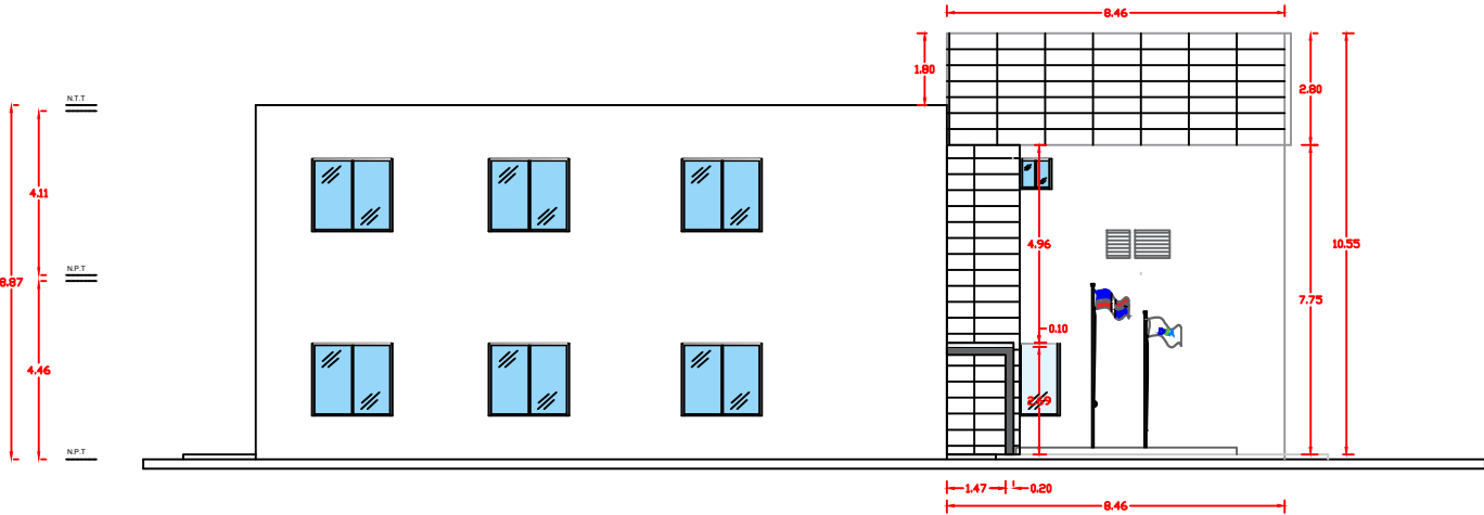
PROPUESTA DE FACHADA DIMENSIONADA ELEVACION LATERAL IZQ.
