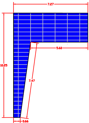
DETALLE DE PROPUESTA DE FACHADA ELEVACION LATERAL DER.
