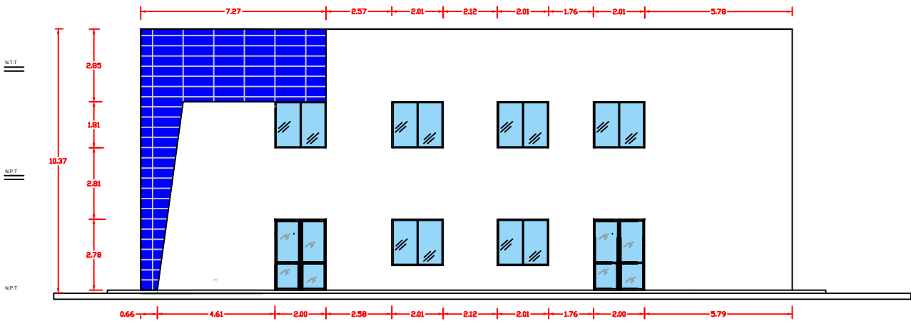
PROPUESTA DE FACHADA DIMENSIONADA ELEVACION LATERAL DER.
