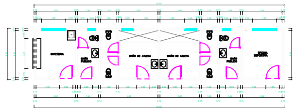
PLANTA ARQ. Y DIM. AREA DE SERVICIOS
