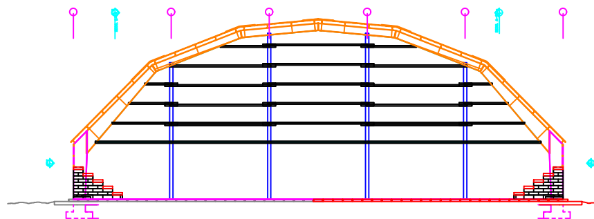
2 SECCION 6-7 A-03 Sin escalar
