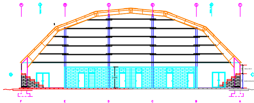
2 SECCION 3-4 A-02 Sin escalar
