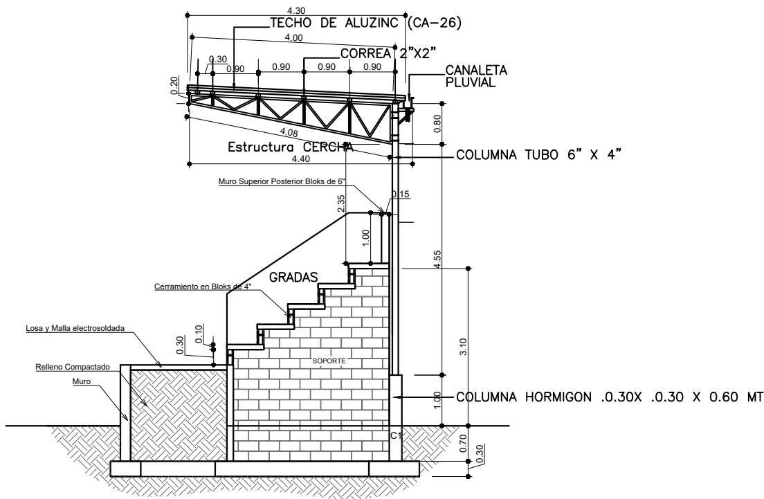
1 SECCION TECHADO DE GRADERIA A-03 ESC.: 1:50
