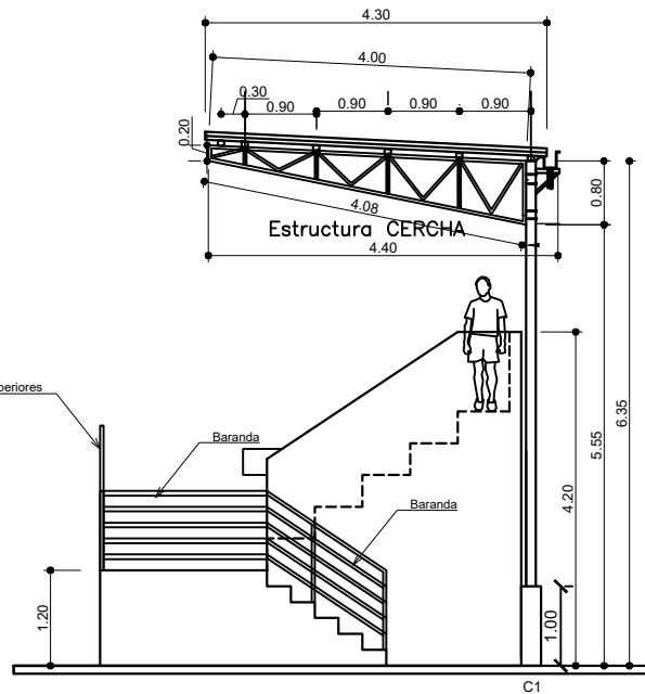
1 ELEVACION LATERAL DERECHA DE GRADERIA A-03 ESC.: 1:50
