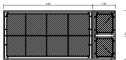
1 DETALLE DE PUERTA CORREDIZA A-03 ESC.: 1:50
