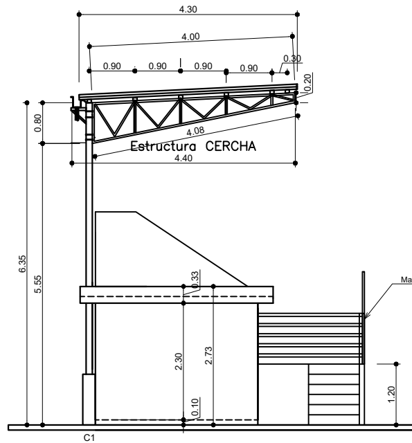
1 ELEVACION LATERAL IZQUIERDA DE GRADERIA A-03 ESC.: 1:50
