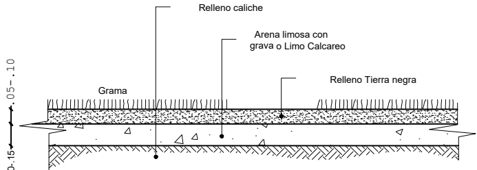
Det. Trreno Cuadro Int. y jardines (no incluye media luna)
