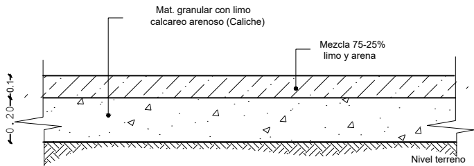
Det. Terreno Media Luna
