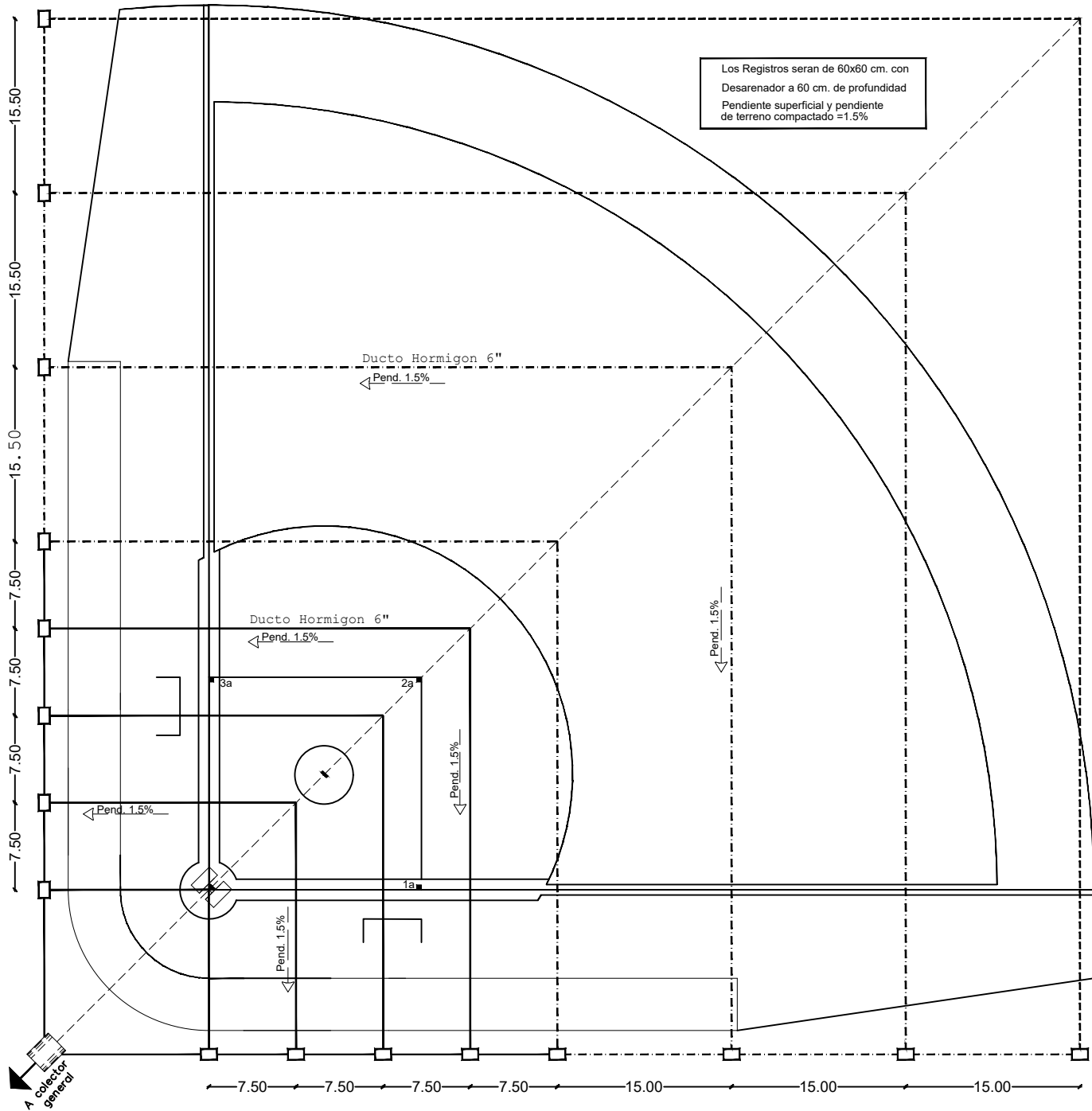
PLANTA DRENADO CAMPO BEISBOL
