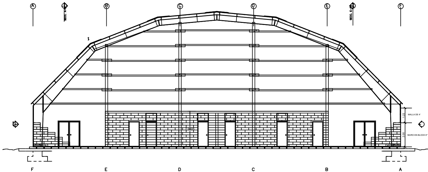
2 SECCION 3-4 A-02 Sin Escala
