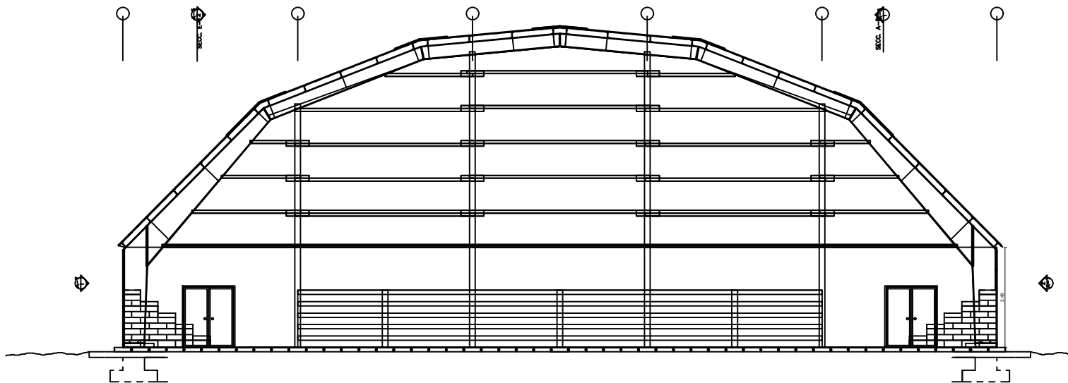
2 SECCION 6-7 A-03 Sin Escala
