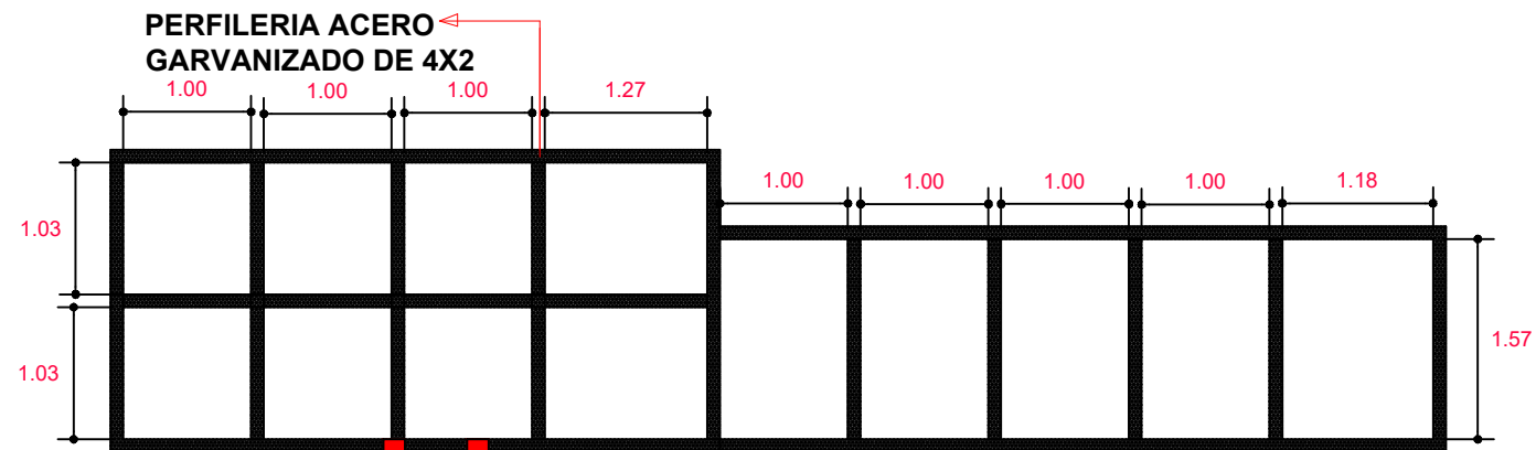
DETALLE EN PLANTA DE LA PERFILERIA METALICA PARA TECHO DE POLICARBONATO
