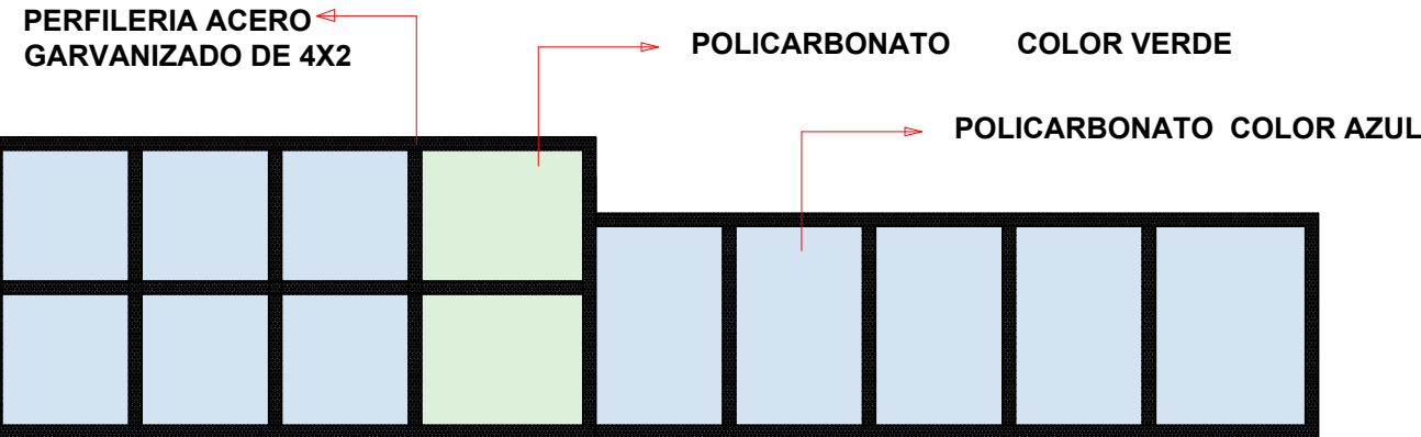
DETALLE EN PLANTA DE LA PERFILERIA METALICA PARA TECHO DE POLICARBONATO
