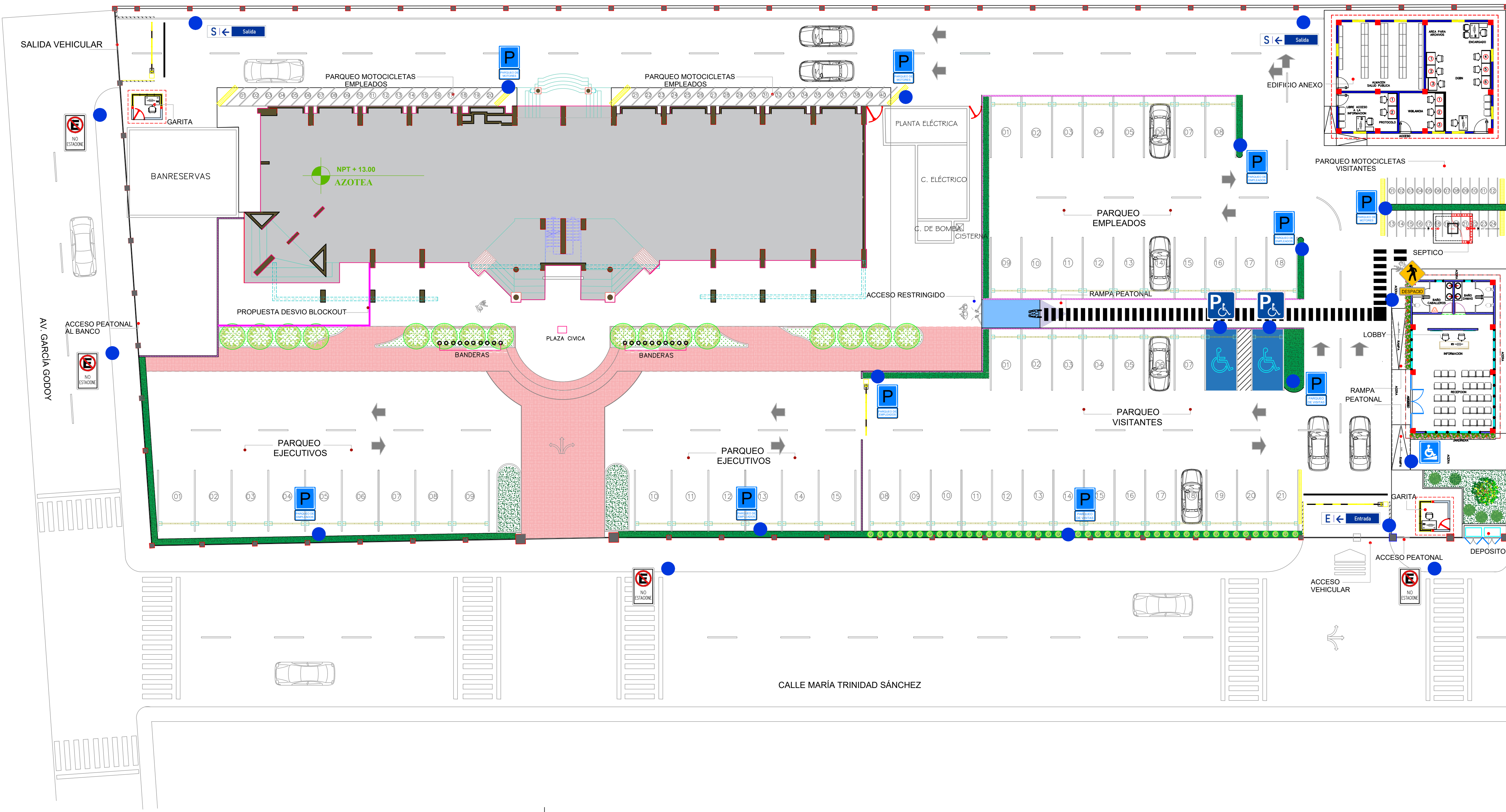
PLANTA DE SEÑALIZACION VIAL ESCALA: 1:50
