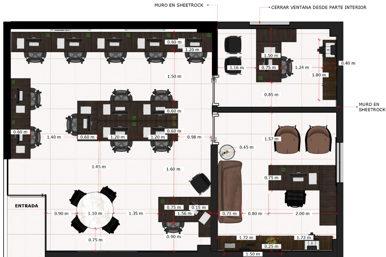
PLANTA DIMENSIONADA
