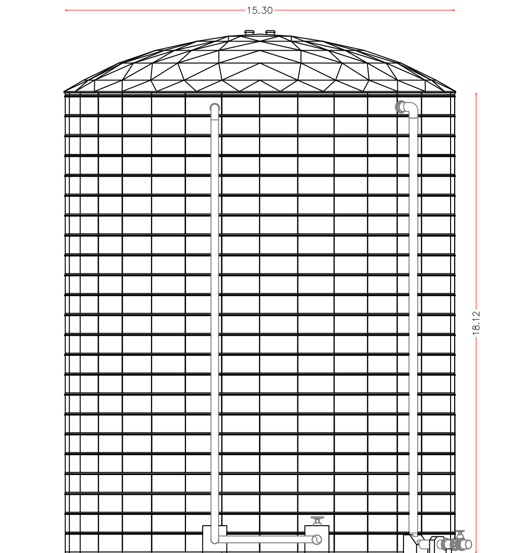
ELEVACION TANQUE PROPUESTO
