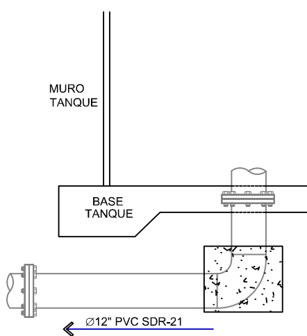
DETALLE SALIDA TANQUE
