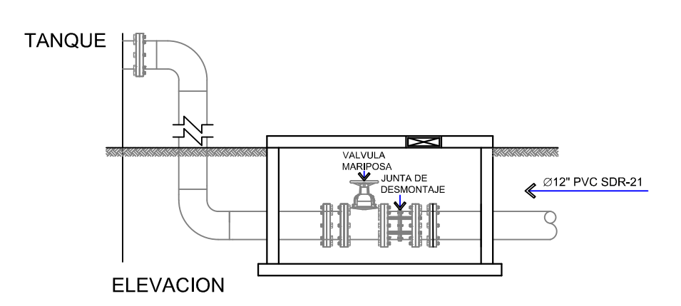
ELEVACION
