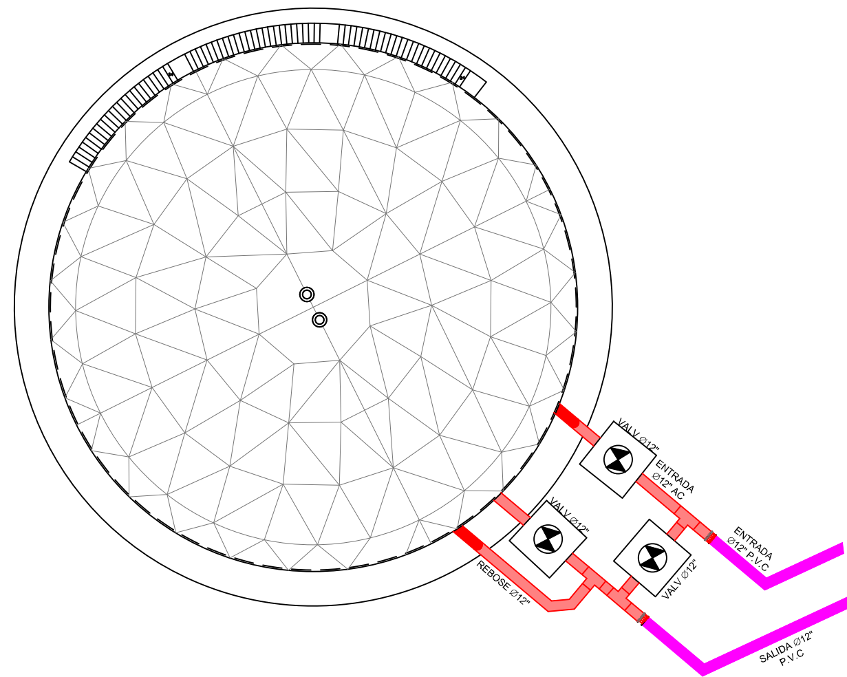
PLANTA TANQUE PROPUESTO
