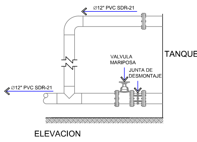
ELEVACION
