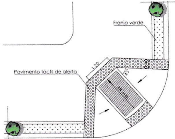
Rampa de esquina
