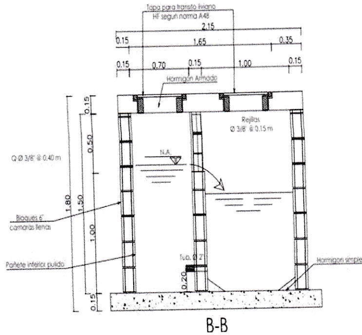
Imbornal de una (1) parrilla
