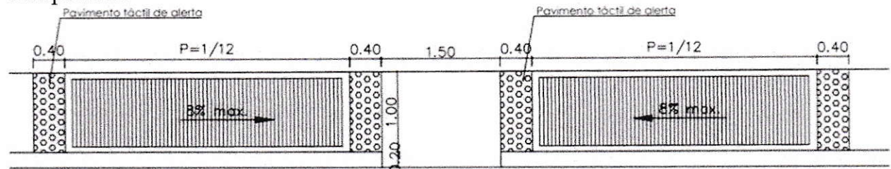
Rampa paralela
