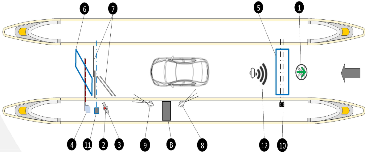
Ilustración 2 Configuración de Vía Mixta Desatendida (VMD)
