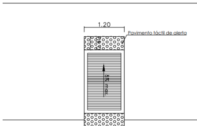
Rampa lineal
