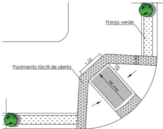
Rampa de esquina
