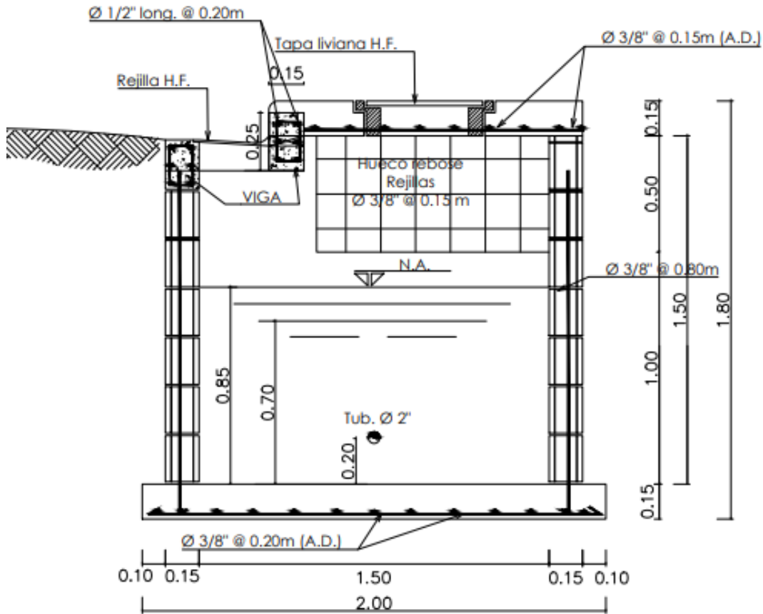
A-A
