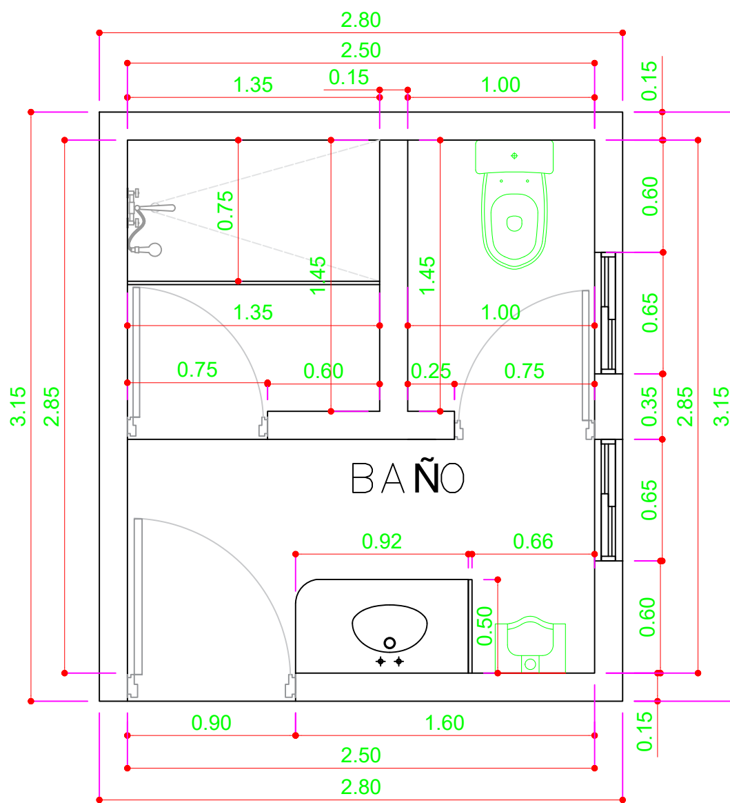
DISTRIBUCIÓN DIMENSIONADA BAÑO
